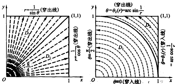
(a) 划分成两个 \theta -型区域 D_1 、 D_2 (b) 用 r=1 线划分成两个 r -型区域
